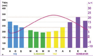
Karadeniz İklimi Yağış Grafiği
