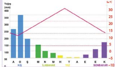
Akdeniz İklimi Yağış Grafiği
