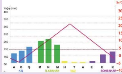
Karasal İklim Yağış Grafiği
